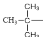
ter-butilo
